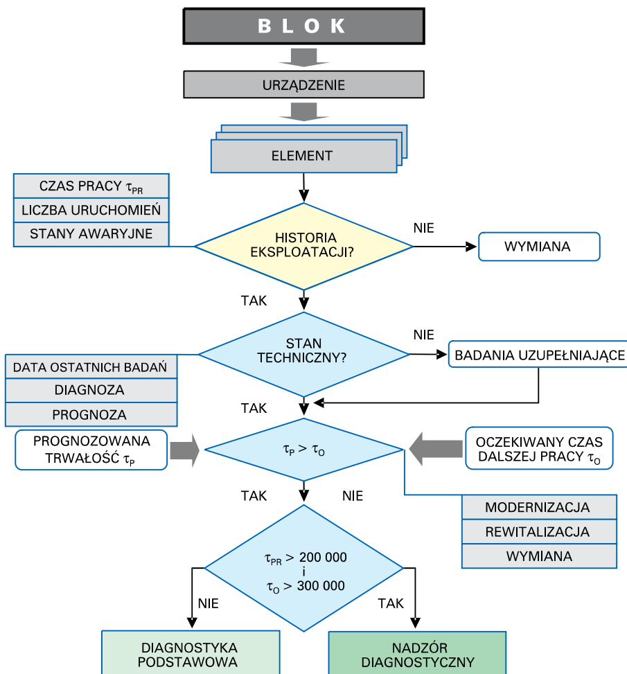
Rys. 2. Wybór rodzaju diagnostyki jako rezultat inwentaryzacji wiedzy o stanie technicznym elementów urządzenia – schemat procesu
